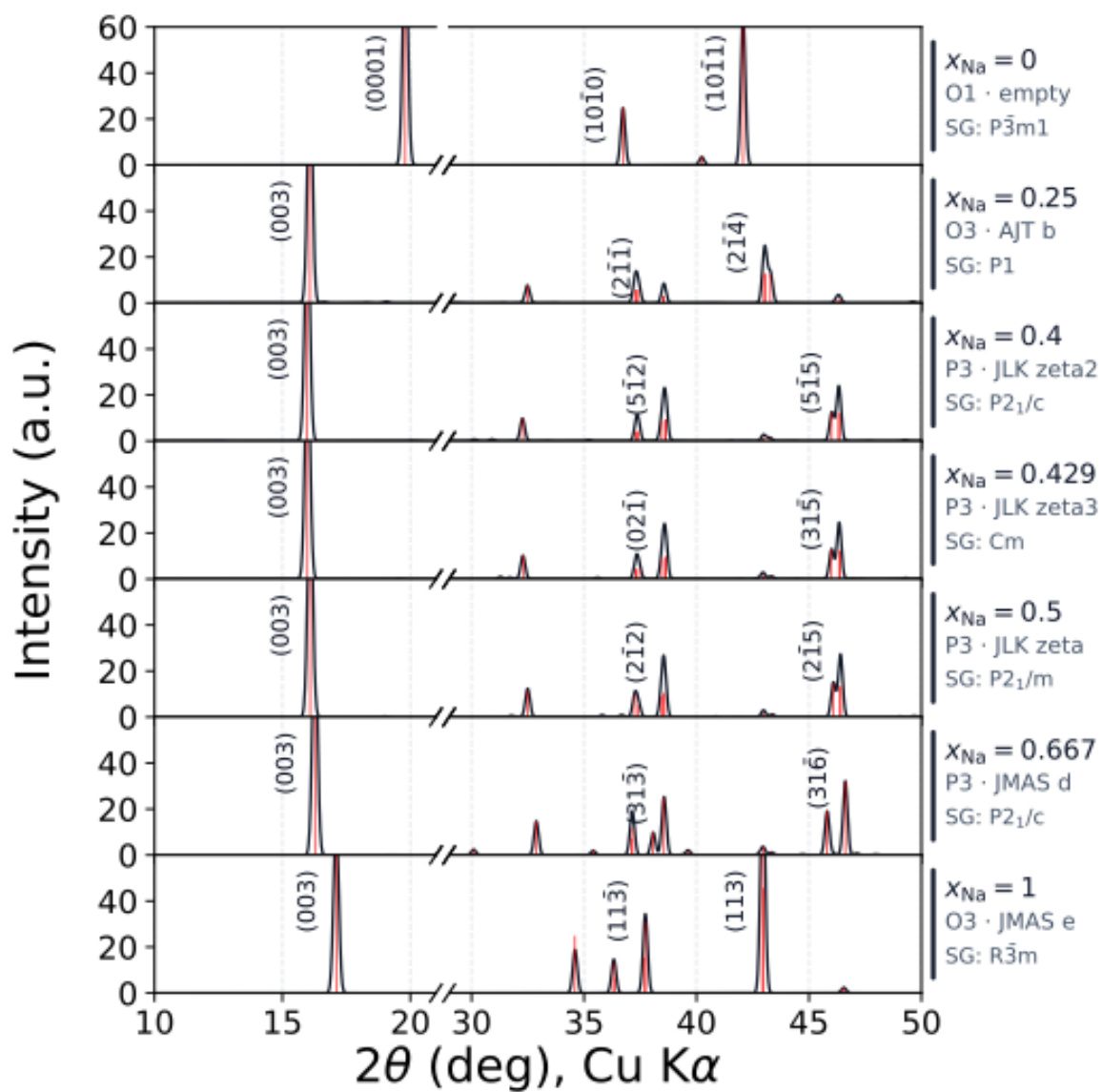
Figure S6 (continued). (d) \text{Na}_x\text{CoO}_2 .
